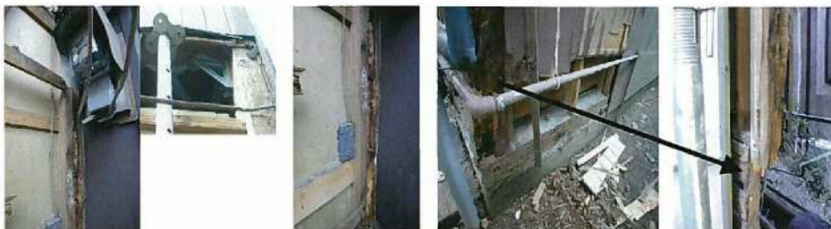
外壁を剥がして中身を見ると、通し柱が腐って無い家に、耐震金物を取り付けられていました。
